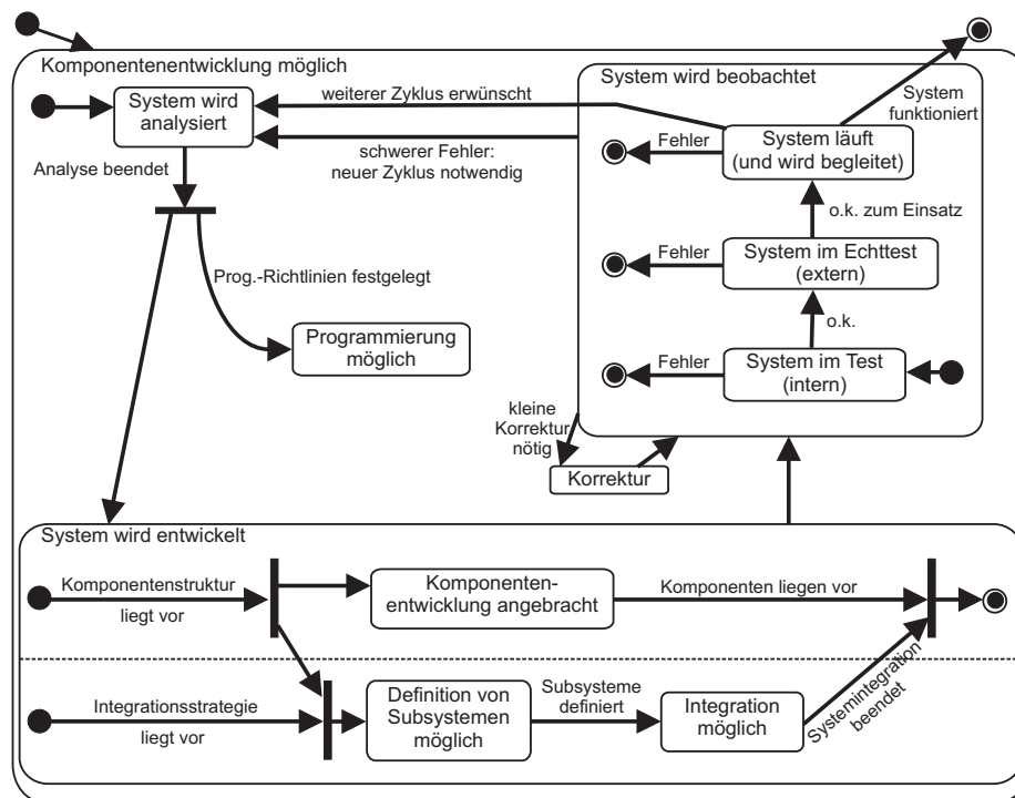
Abbildung 3: Das Zustandsdiagramm der Systemebene
