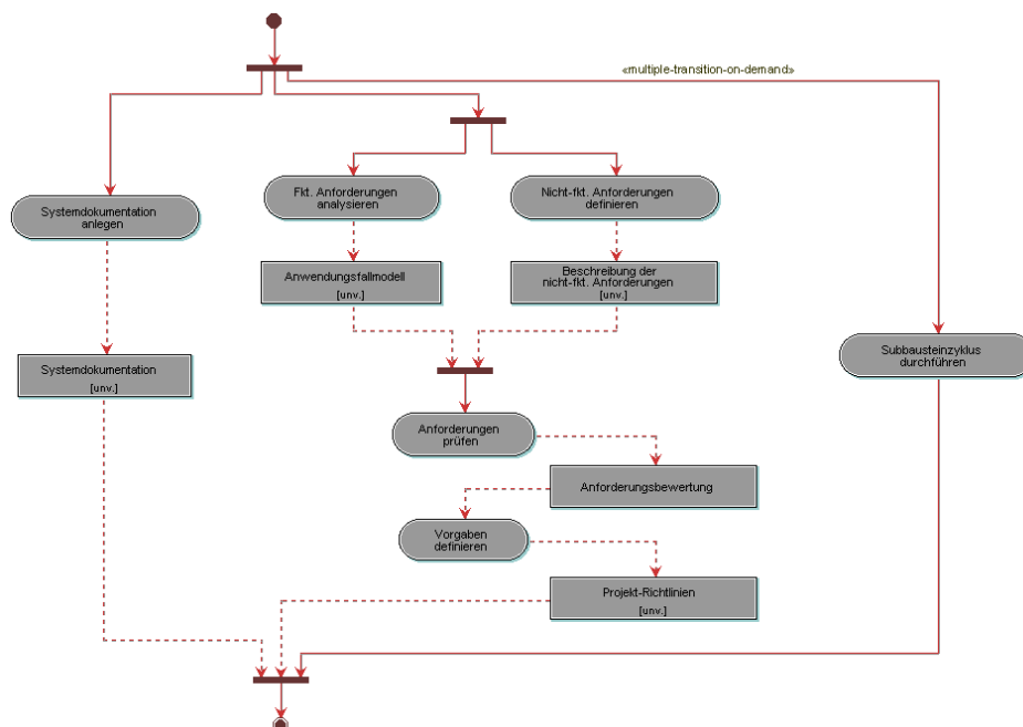
Abbildung 2: Aktivitätsdiagramm der Phase System.Analyse
