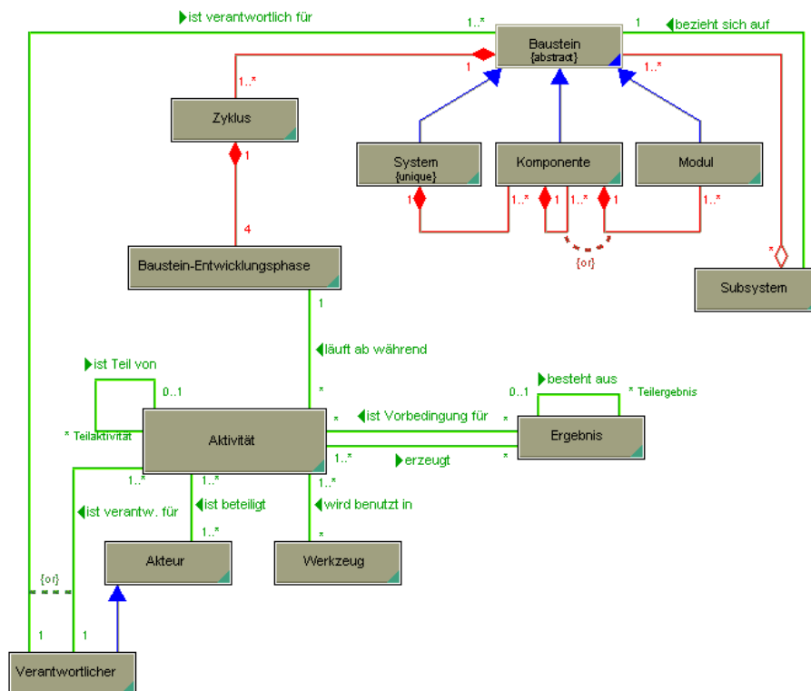
Abbildung 1: Das statische Metamodell als Klassendiagramm
